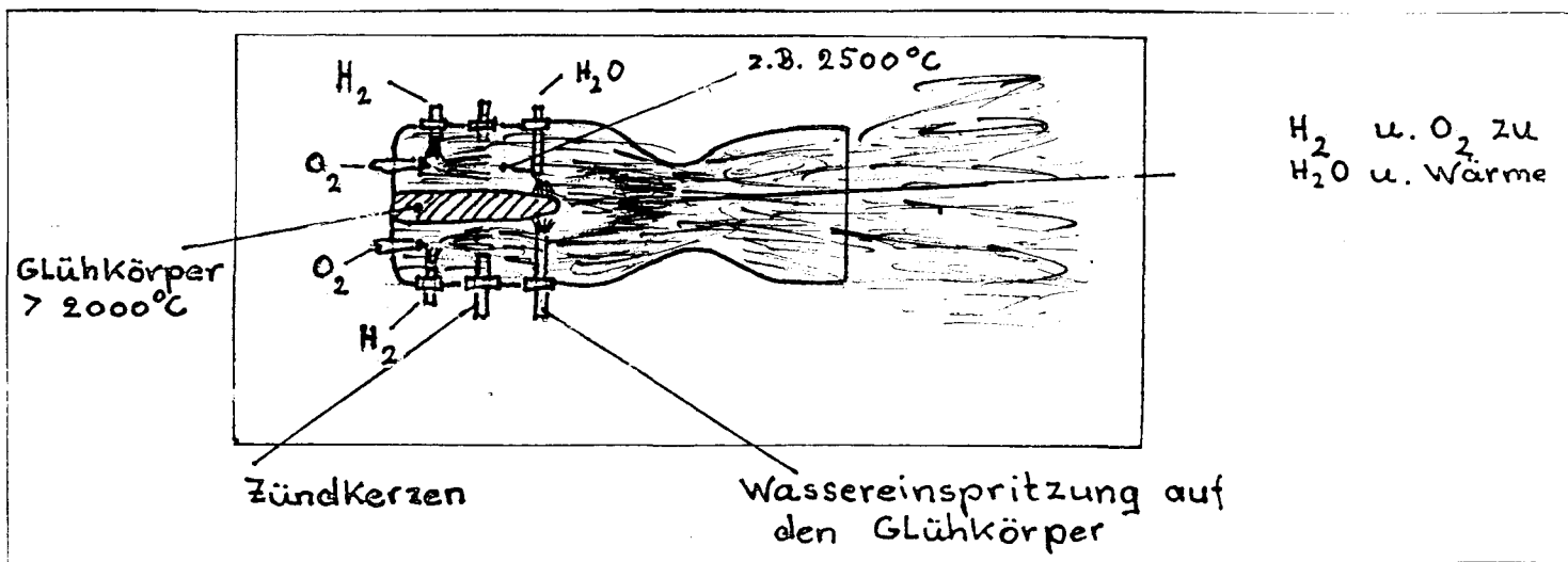
Abbildung 7 Raketen-Brennkammer
