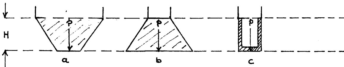
Abbildung 16a – c Das hydrostatische Paradoxon
