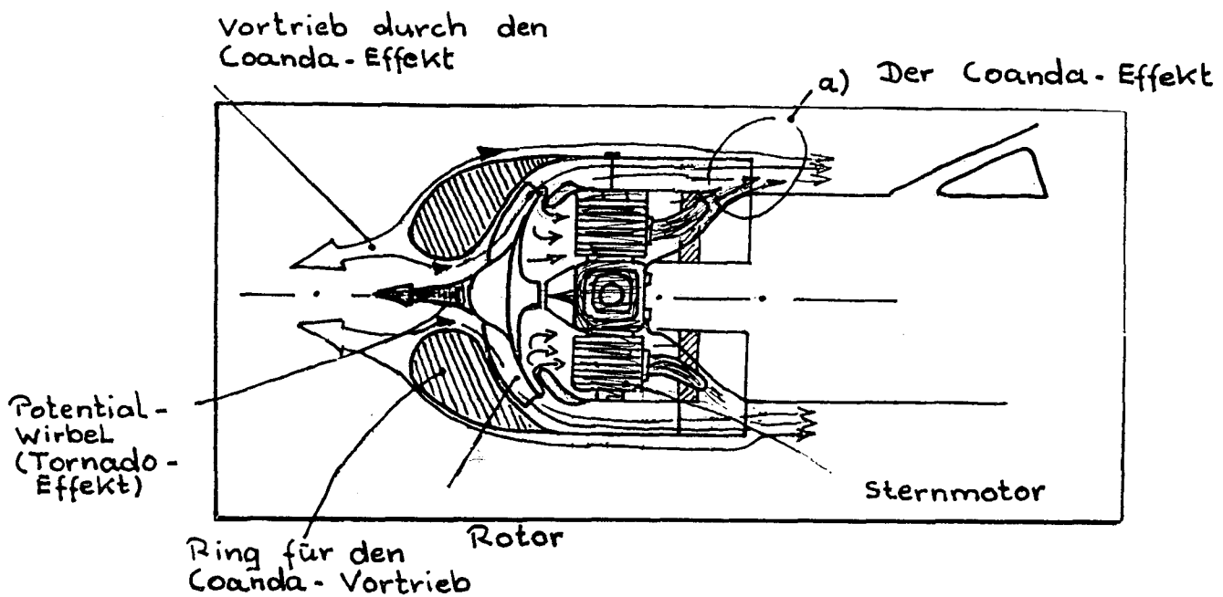
Abbildung 2 Antriebsmechanismus
