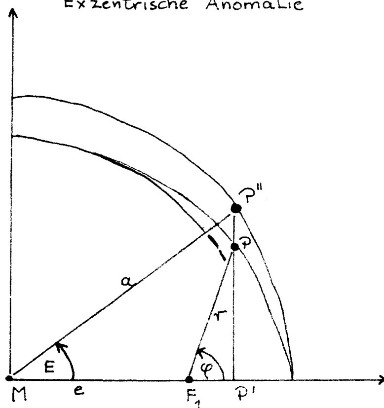
Abbildung 4 Exzentrische Anomalie
