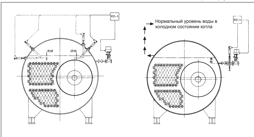
Пример установки
